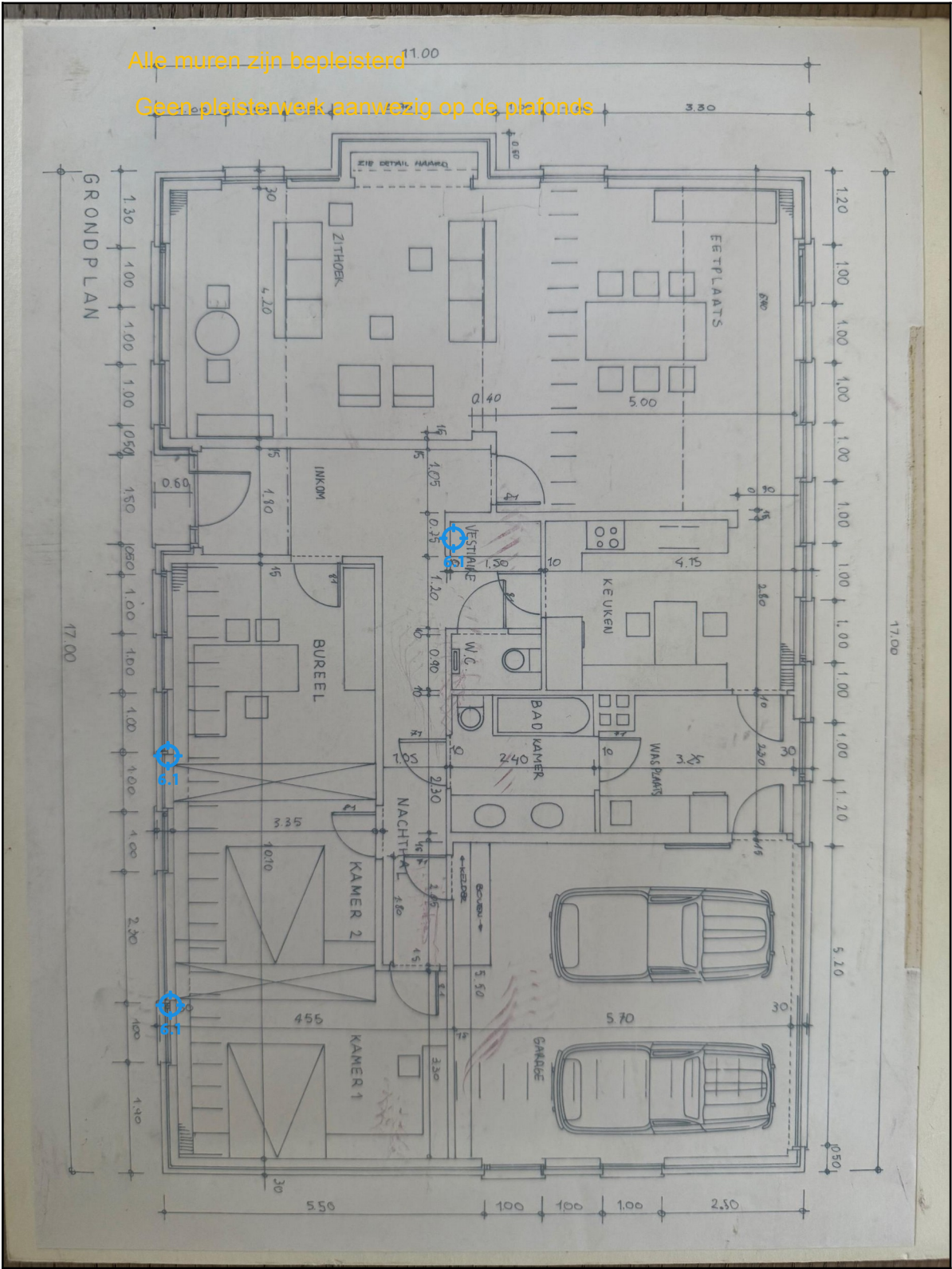
Legende van plan 1.1: Plan V0 zonder uitbouw
